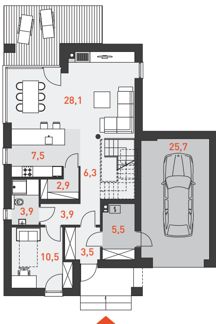
RZUT PARTERU 66,6 m 2
